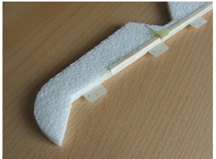
Vyříznout zářezy pro panty. Vyříznout zárez pro ovládací páku a páku zalepit.
